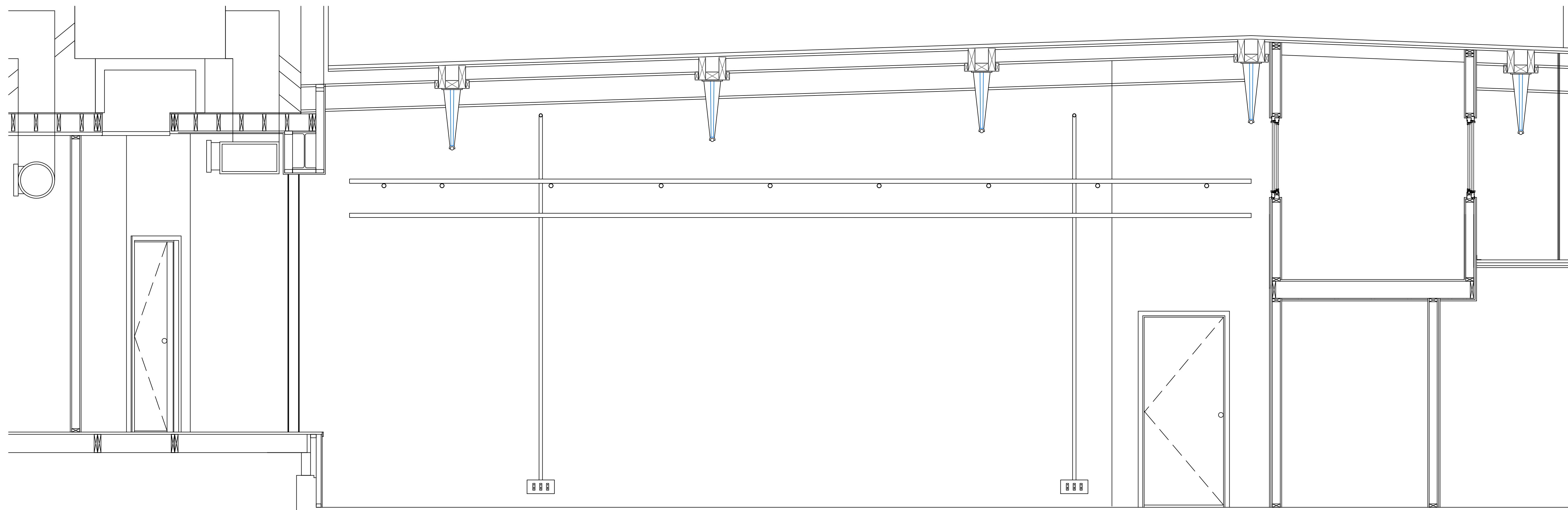
1 Longitudinal Section
